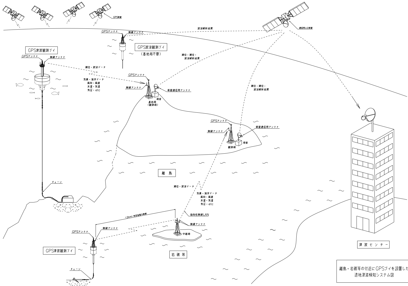
図 2.2.2 離島・岩礁等の付近にGPSブイを設置した遠地津波検知システム図
